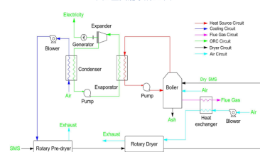
圖3 生質能發電系統創新架構圖(Patent pending)
