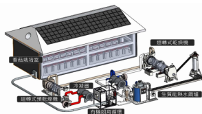
圖2 生質能系統3D圖
