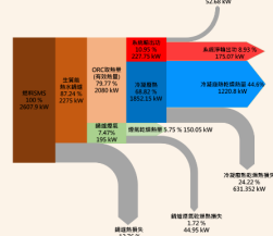
圖4 生質能系統燃料能轉換之能量流動(Energy flow)
